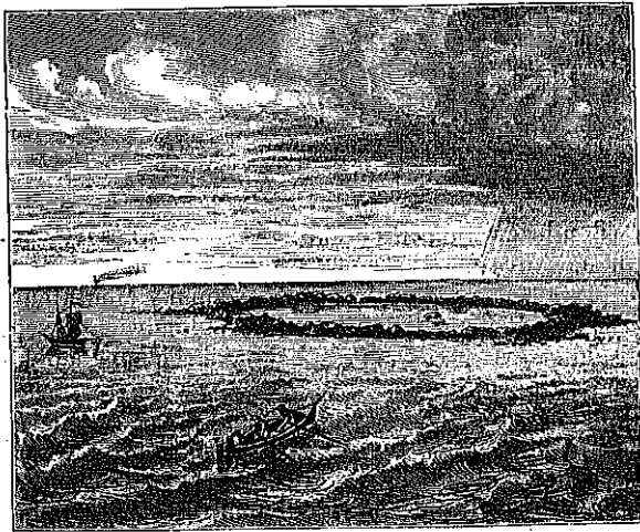
Koralový ostrov kruhový s jezerem či atolem.
