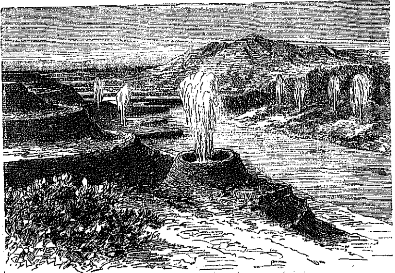
Přirozené vodotrysky na Novém Seelandě.
